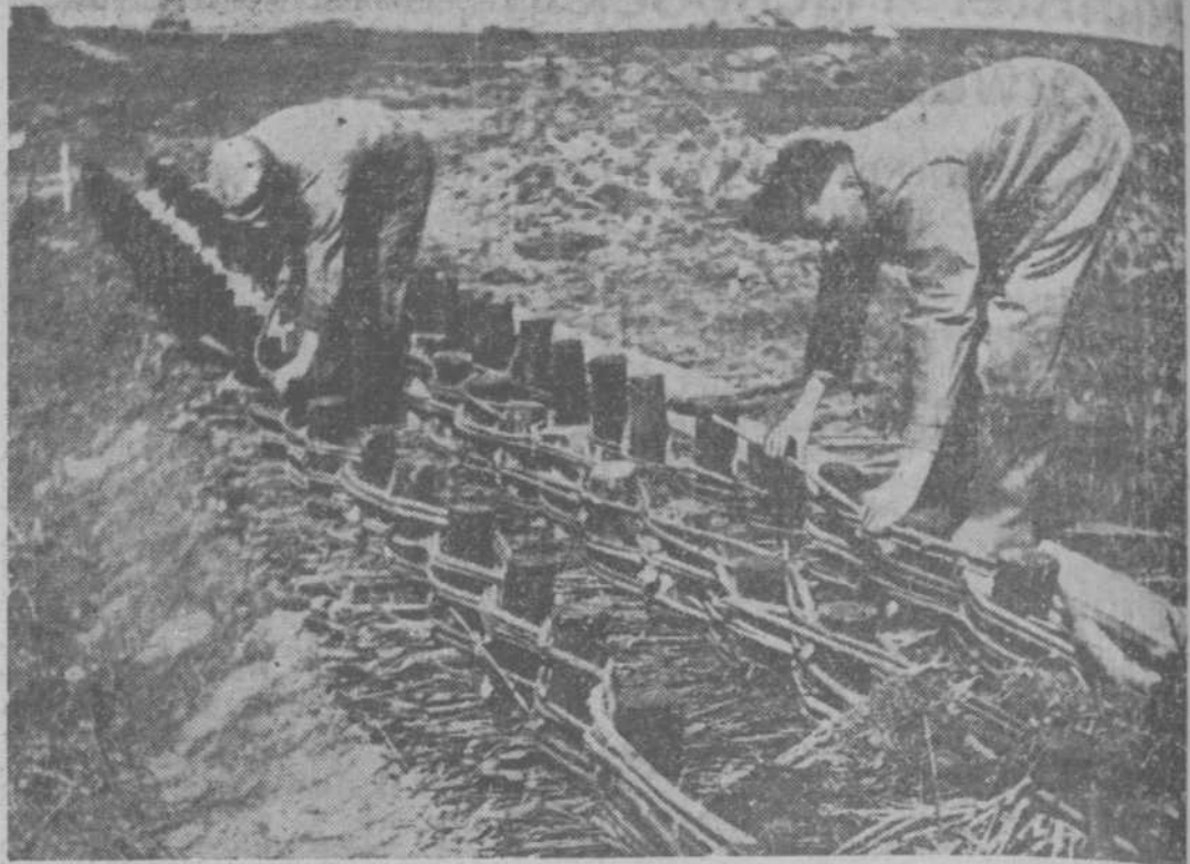
Geen schoeiing van beton of ijzeren balken. — Wie niet sterk is moet slim zijn, zegt het spreekwoord. De oplossing is gevonden in het vlechten van rijnhout. De ruimten tusschen de drie „vlechtuinen" worden opgevuld met rietzoden. (Pax Holland)
